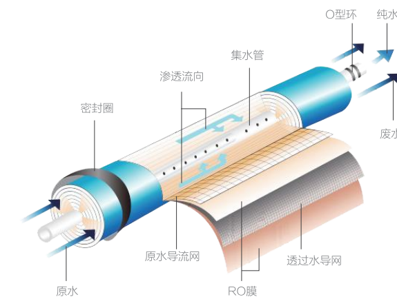
RO模式图
