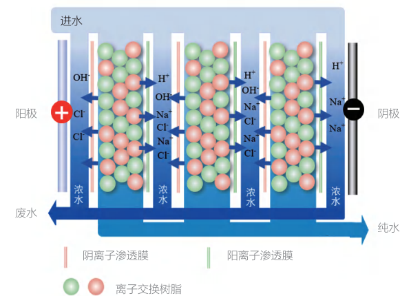
EDI原理图
