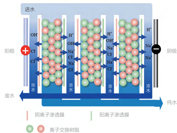
EDI原理图
